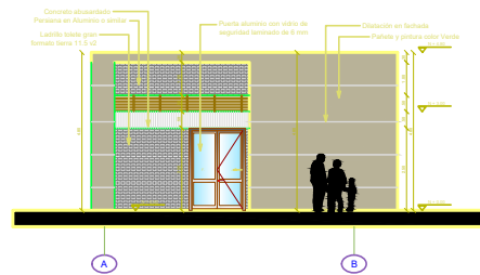
FACHADA LATERAL IZQUIERDA ESC. 1:75
