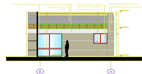
LATERAL DERECHA ESC. 1:75
