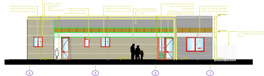
FACHADA POSTERIOR ESC. 1:125
